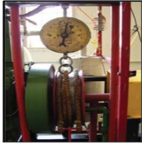
b. Rope Brake Dynamometer
